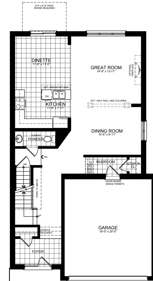
ELEV. A
