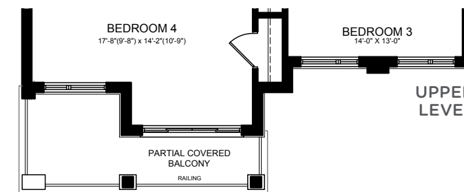
ELEV. C
