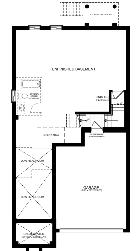
ELEV. A
