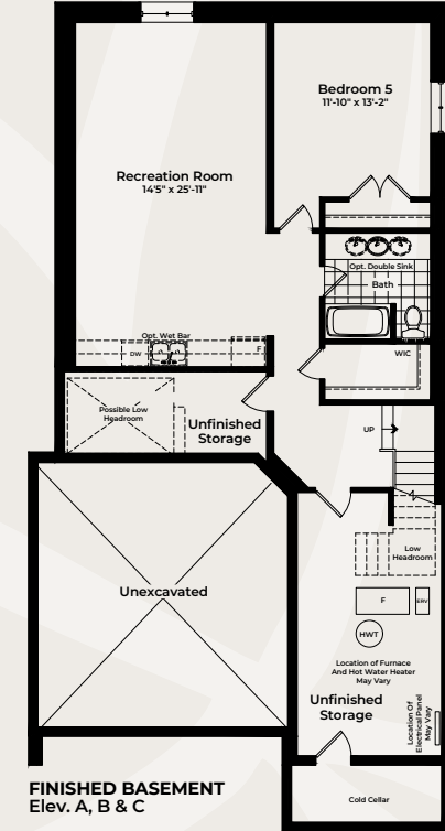
ELEV. C 3,941 SQ.FT.
